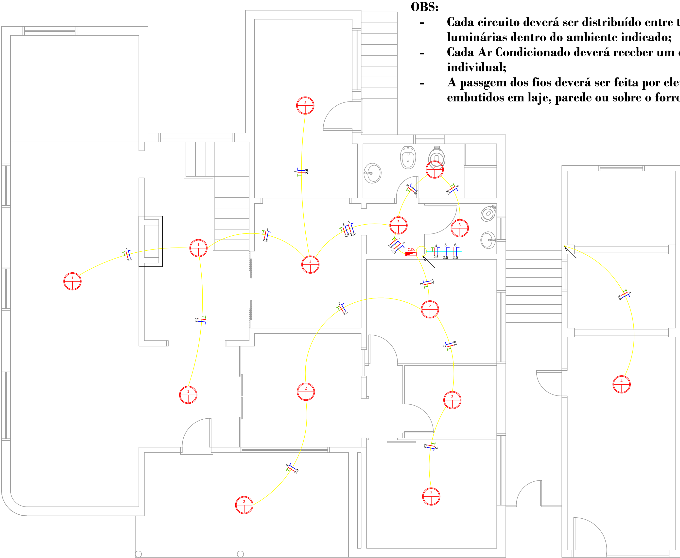
DISTRIBUIÇÃO DOS CIRCUITOS - TÉRREO
